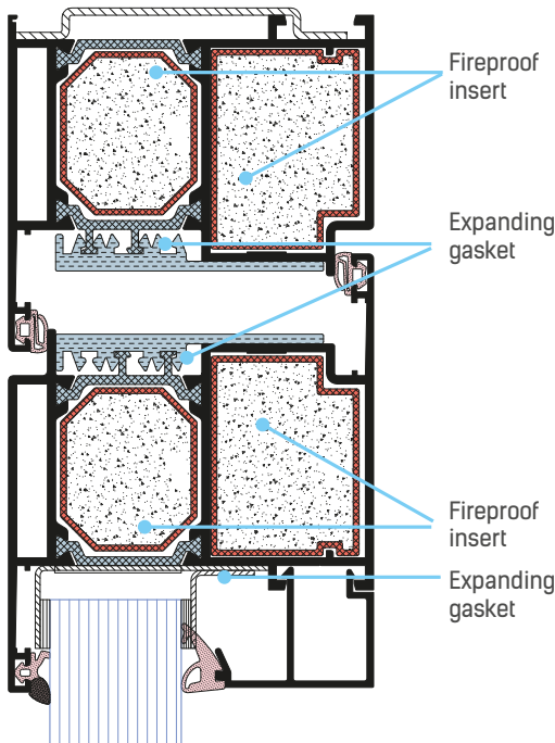
EI60 class door
